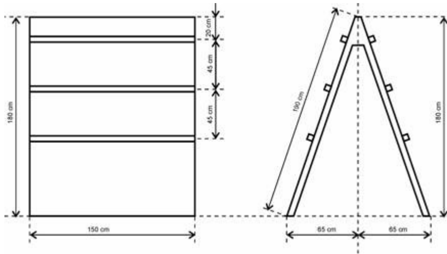
Obrázek č. 5 :Šikmá stěna - bariéra Pohled zepředu - Pohled z boku
